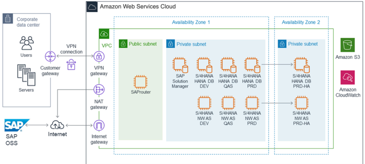
图 3：SAP 全能架构Amazon
