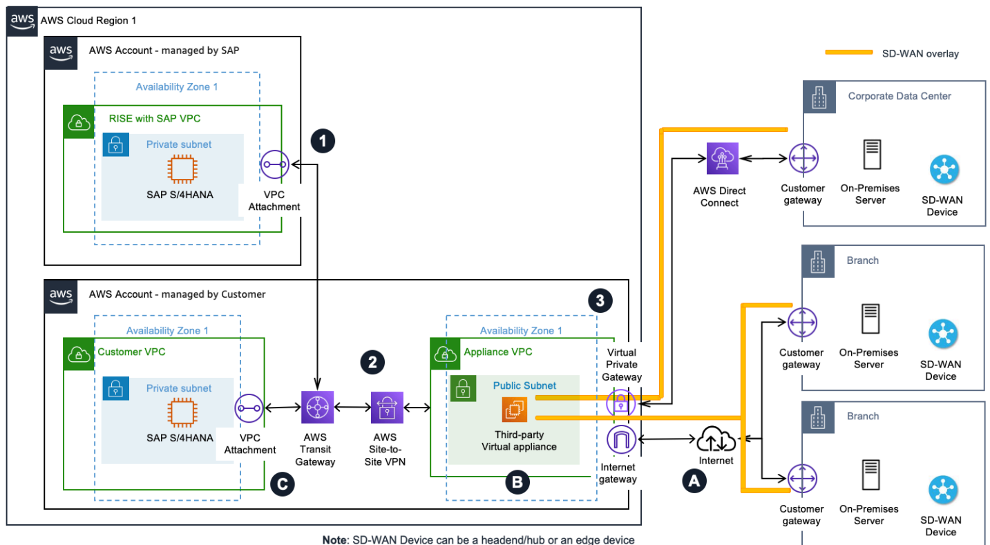
模式 B-2：与 Amazon Site-to-Site VPN Amazon 集成的 SD-WAN 设备
