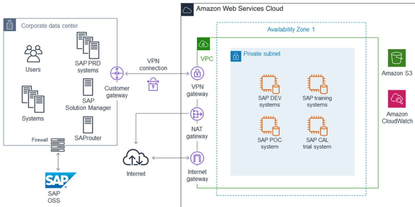
图 4：SAP 混合 Amazon 架构
