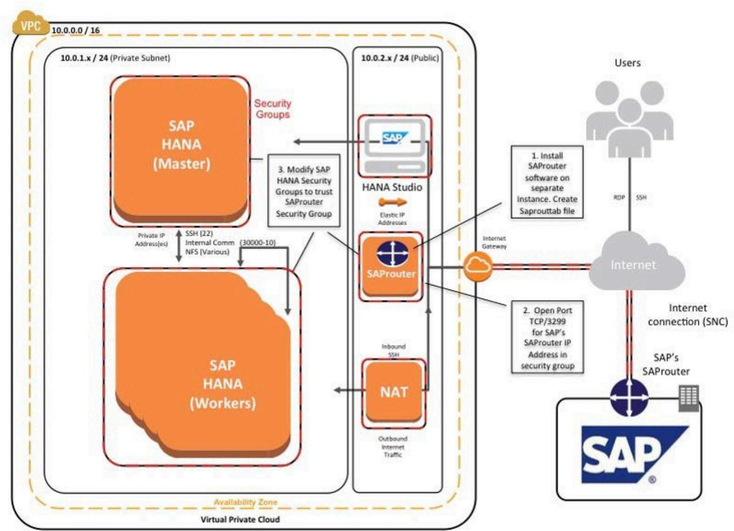
图 13：在 Amazon 云端使用 SAProuter 的支持连接
