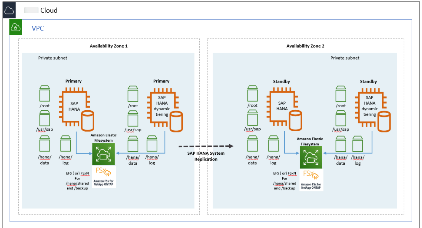
图 2：开启 SAP HANA 动态分层 Amazon（多可用区）
