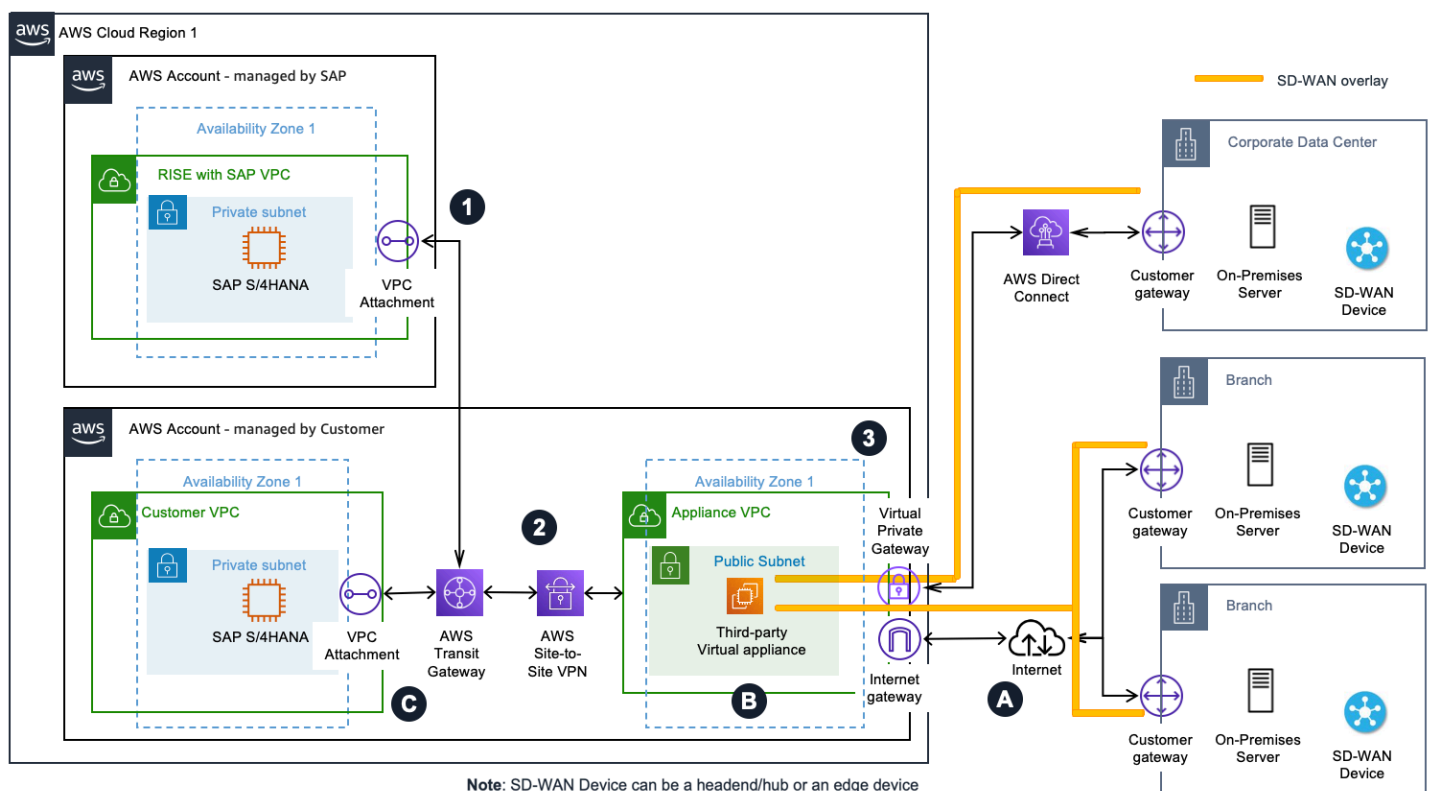
模式 B-2：与 VPN 集成的 SD-WAN 设备 Amazon Amazon Site-to-Site
