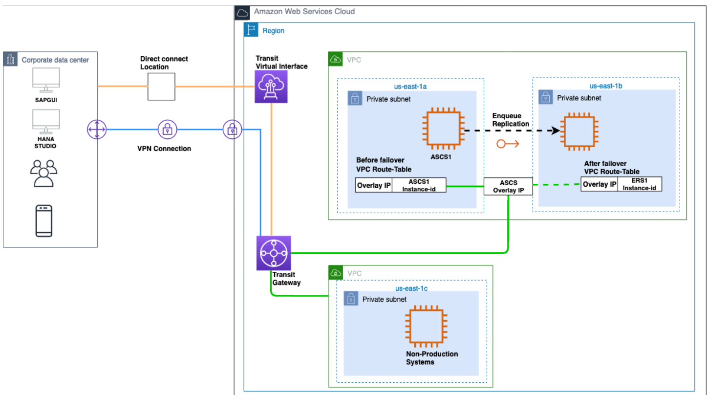
图 1：使用叠加 IP 地址设置 Amazon Transit Gateway
