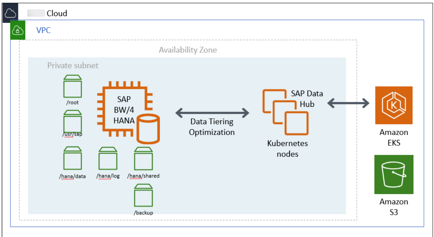
图 8：带有 BW4 /HANA 的亚马逊 EKS 上的 SAP 数据中心
