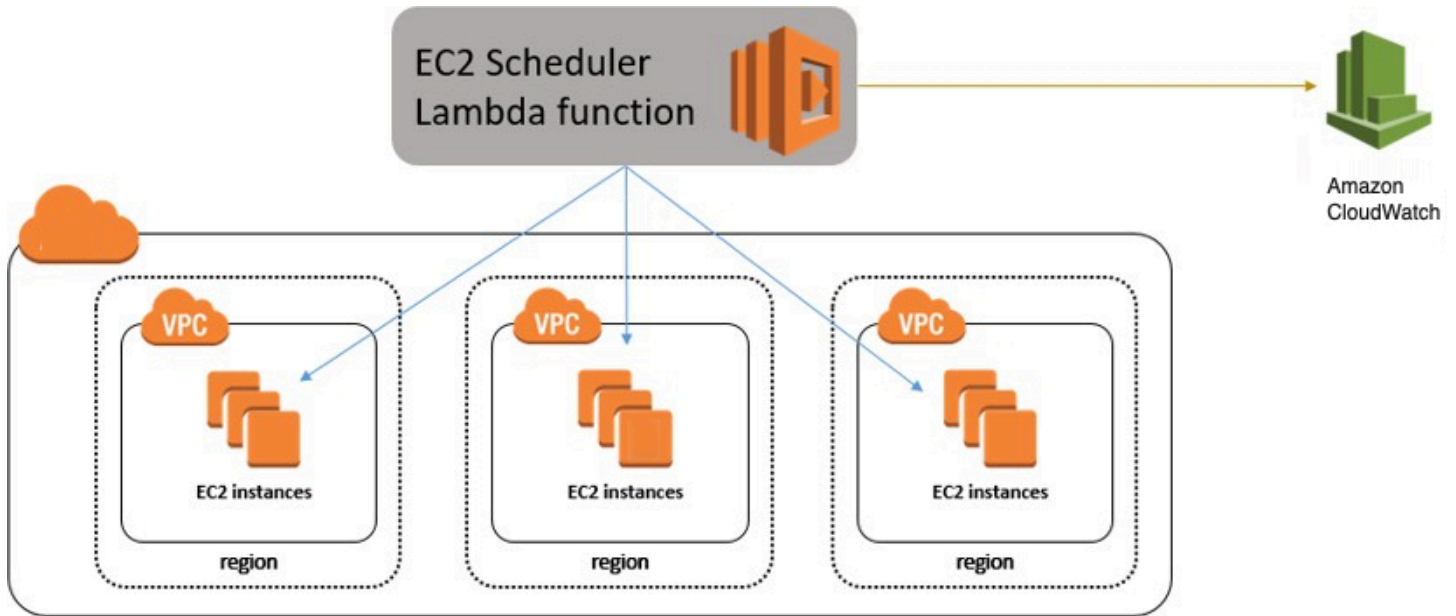
图 1：EC2 调度程序
