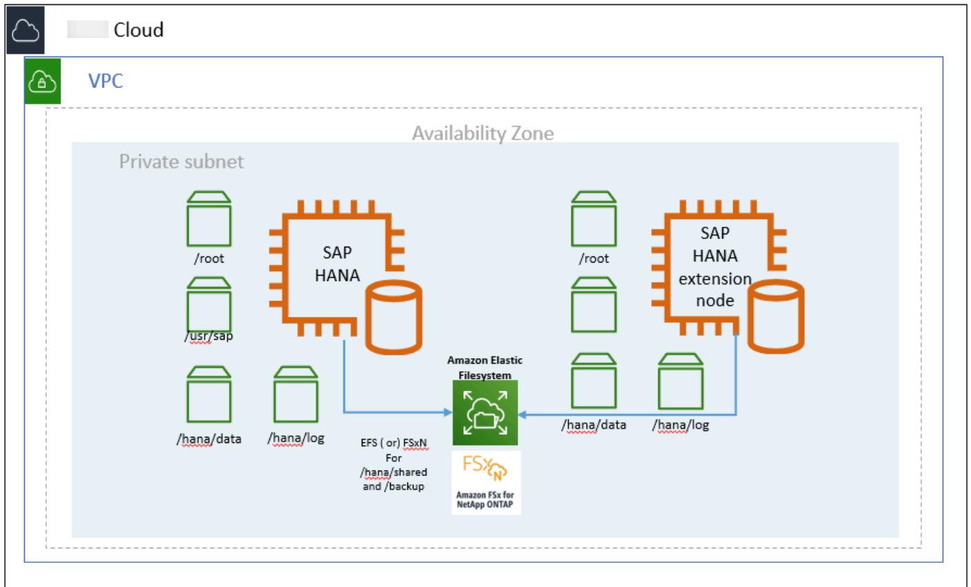
图 3 : 开启的 SAP HANA 扩展节点 Amazon
